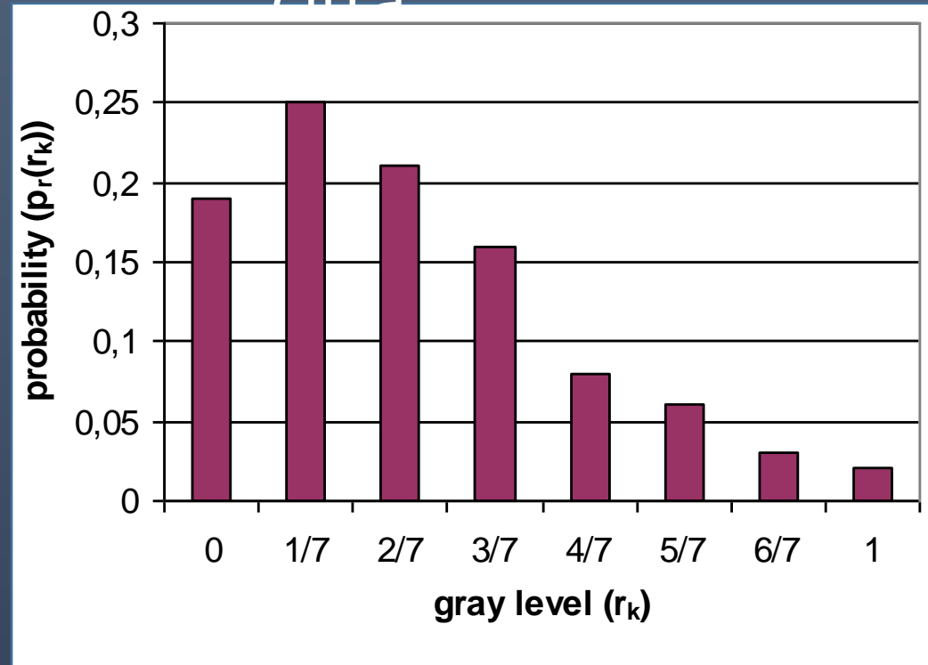
Histogram citra:
